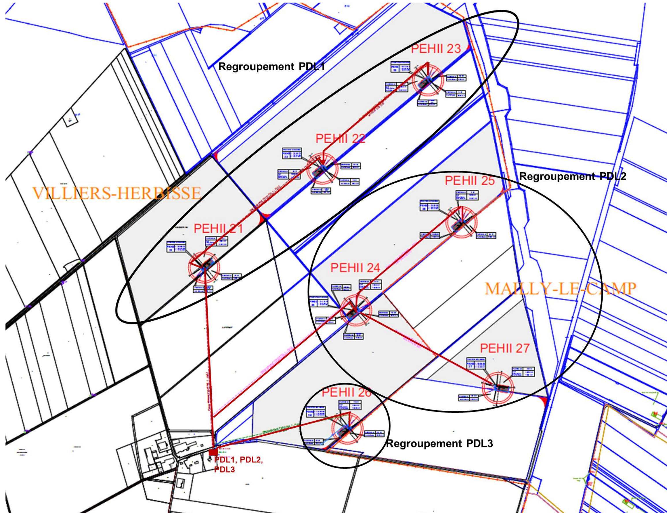
Carte 12 : Extrait du plan d'implantation des postes de livraison et réseaux inter-éoliens – Source : Plan masse général
