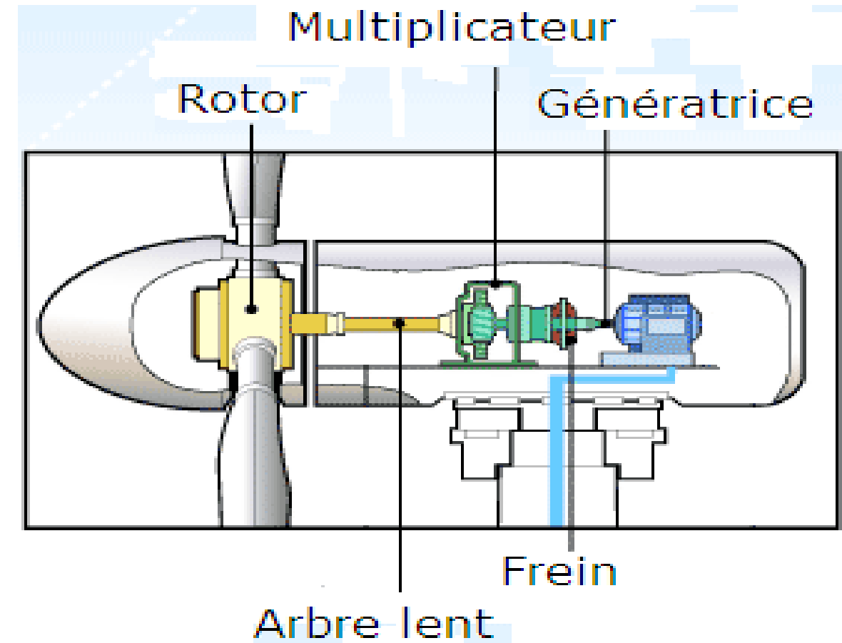
Figure 8: Schéma simplifié de la chaîne cinématique
