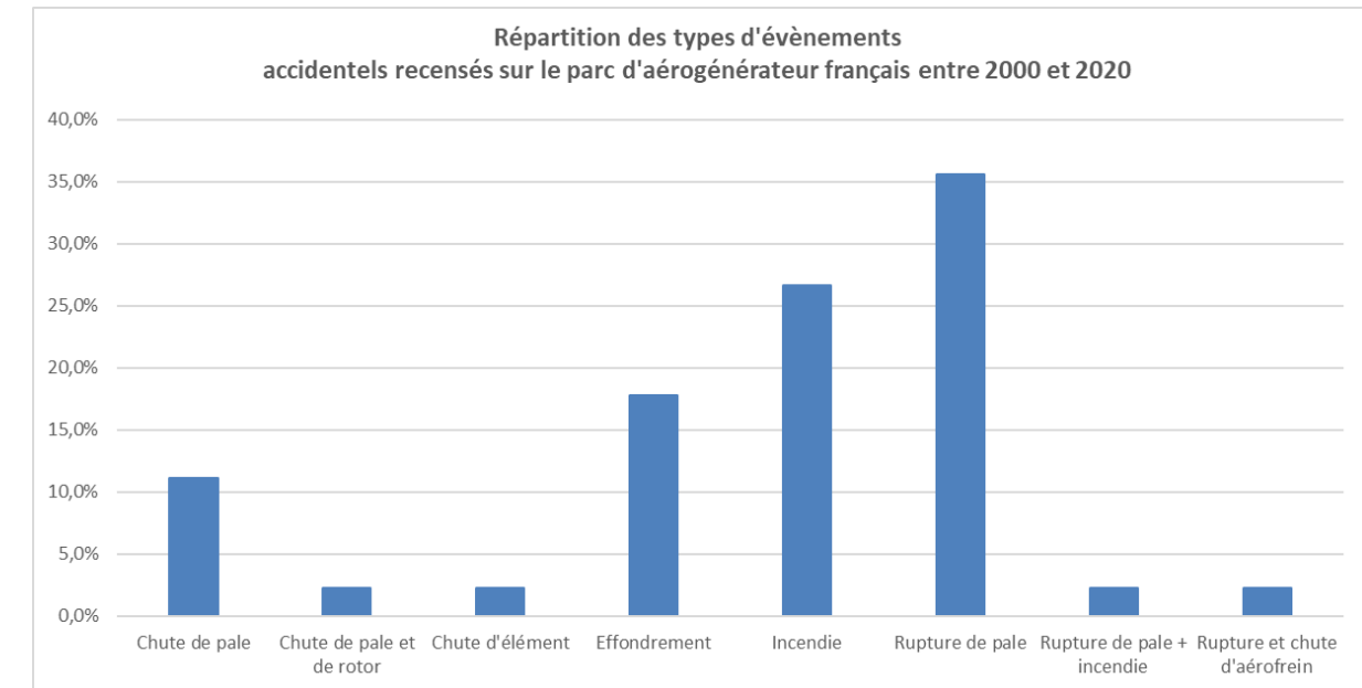
Figure 11 : Répartition des événements accidentels sur le parc d'aérogénérateurs français entre 2000 et 2020
